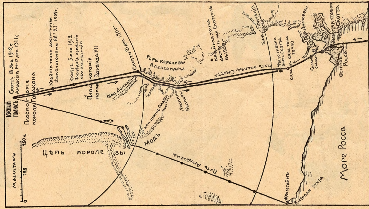
Схема движенія отряда кап. Скотта къ южному полюсу и его обратнаго пути.
